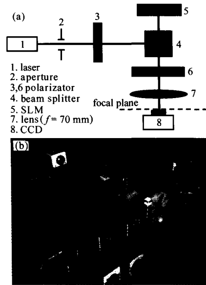
图 4 光束偏转实验装置图
